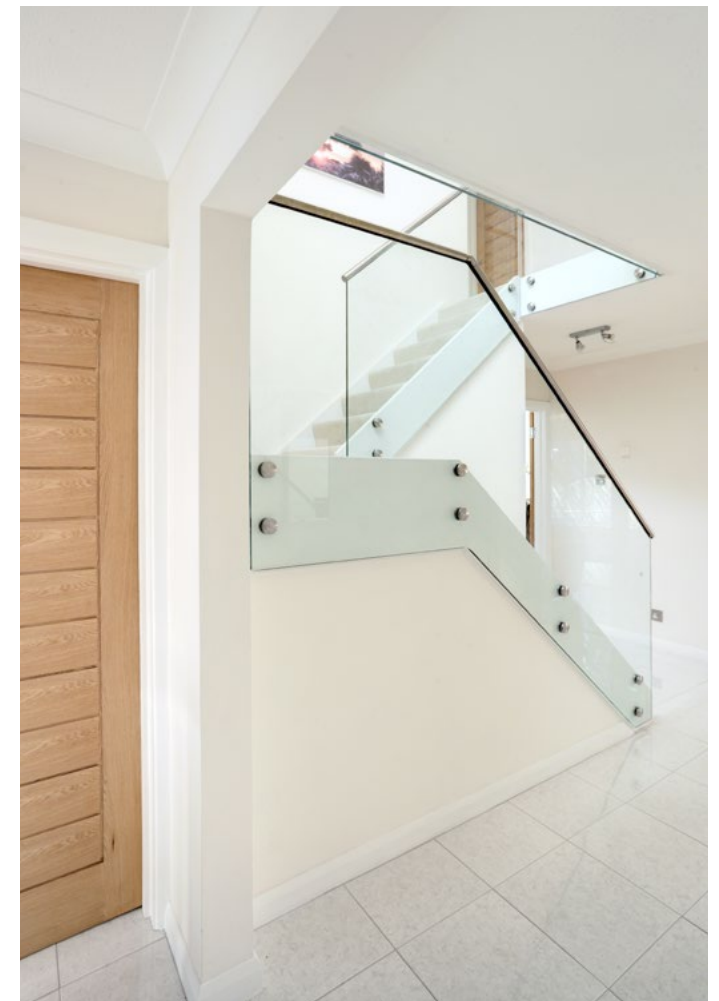
→ Punktfäste Easy Glass® Mod 0745 Foto: Q-Railing
